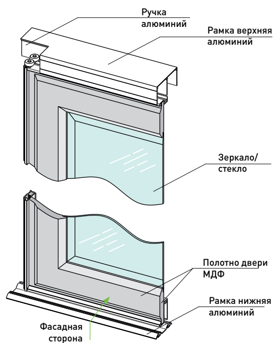
Схема односторонней двери
