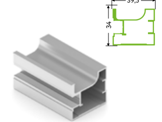
FA0413.VP540 Профиль вертикальный FUSION Длина – 5,4 м В упаковке 8/6 шт.
