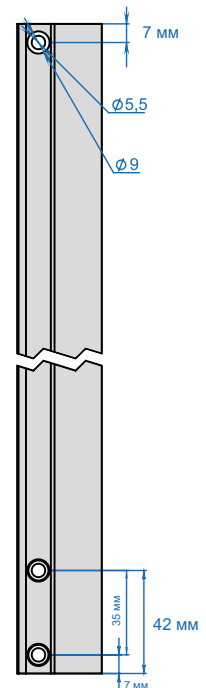
Схема сверления отверстий в профиле вертикальном раздвижной системы
