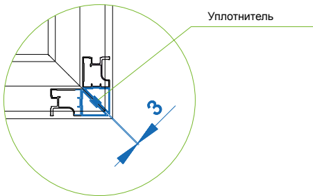
Скос под 45° верхней и нижней направляющей
