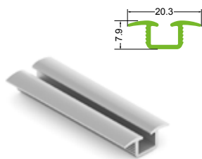
AS0690.VP540 Направляющая врезная однополосная нижняя
