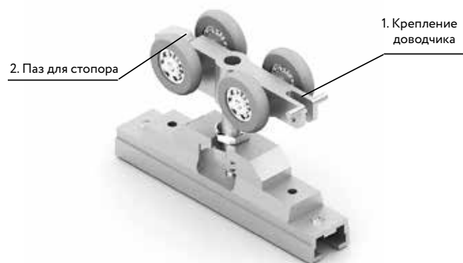
8.2. Установите стопоры.
