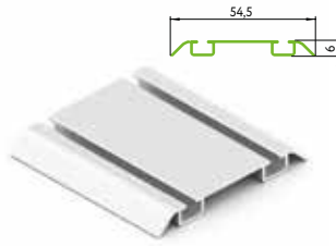
AV0648.VP540 Направляющая двухполосная нижняя
