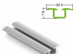
AS0690.VP540 Направляющая врезная однополосная нижняя
