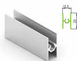
AE0491.VP540 Рамка средняя ЭКО 491
