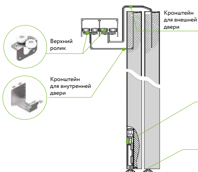
Скрытая установка направляющей верхней
