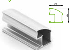
AB0654.VP490 (4,9 м), AB0654.VP540 (5,4 м) Профиль вертикальный Contour
