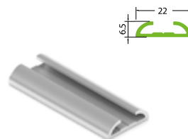
AS0044.VP540 Направляющая распашной двери
