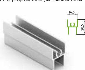
AB0646.VP540 Рамка верхняя
