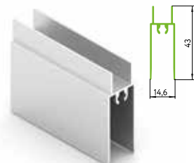
AB0643.VP540 Рамка нижняя
