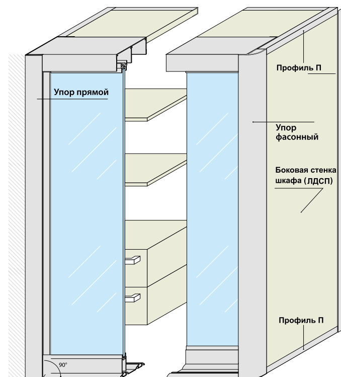
Установка прямого и фасонного упоров
