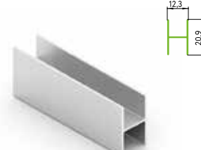
AE0471.VP540 Рамка средняя без самореза
